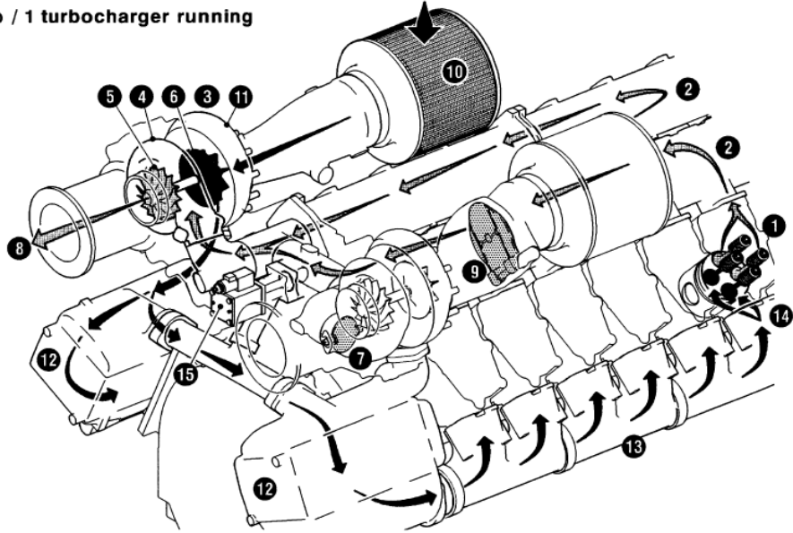
2 ATL in Betrieb / 2 turbochargers running
