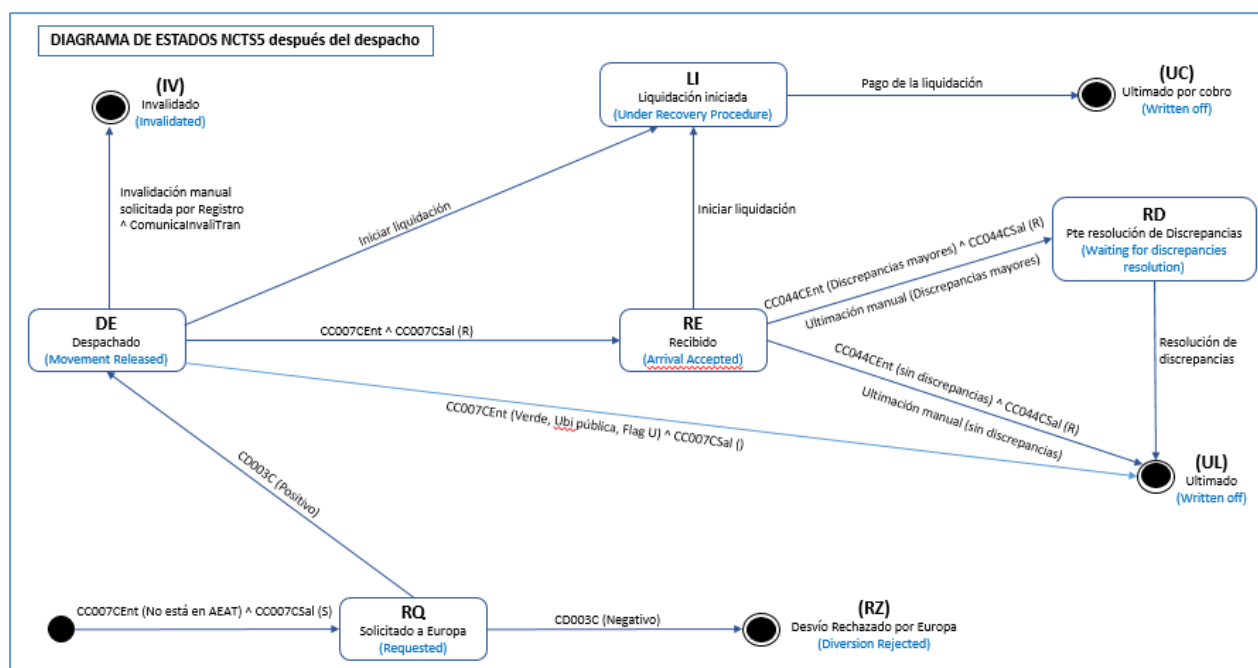
Diagrama de Estados NCTS5 español después del despacho
