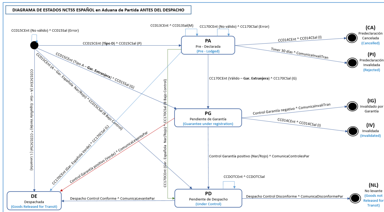
Diagrama de Estados NCTS5 español en Aduana de Partida antes del despacho
